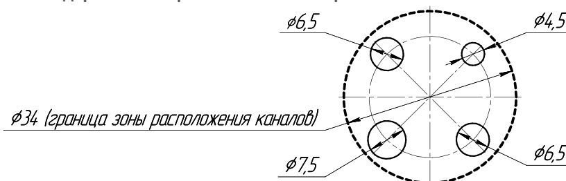
Стандартный набор каналов в блоке сравнения ЭЛЕМЕР-ТК-П150
